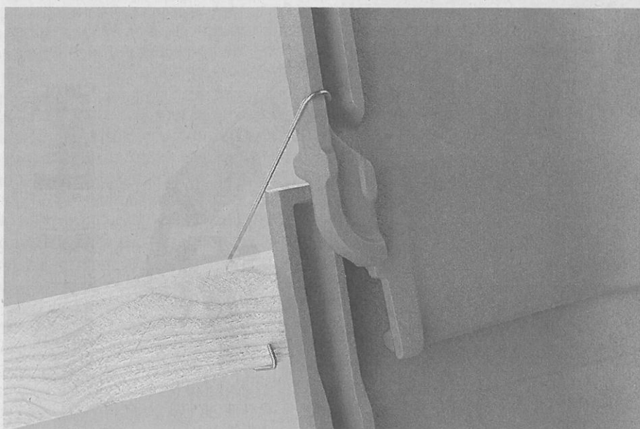
Sitz der Seitenfalzklammer an der Lattung.
