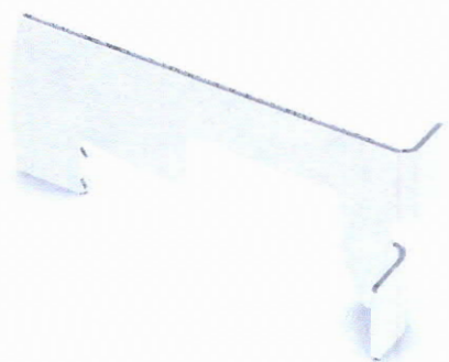
Sturmklammer 425 von FOS für Biberdeckung
