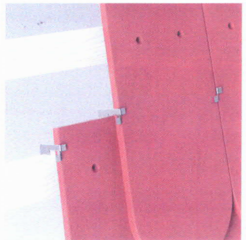
Sturmklammer 425 von FOS für Biberdeckung
